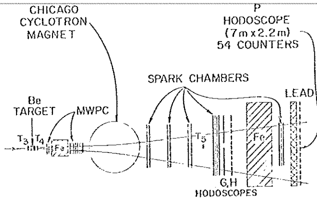
Fig. 1 The Apparatus
